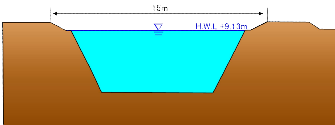
計画横断
