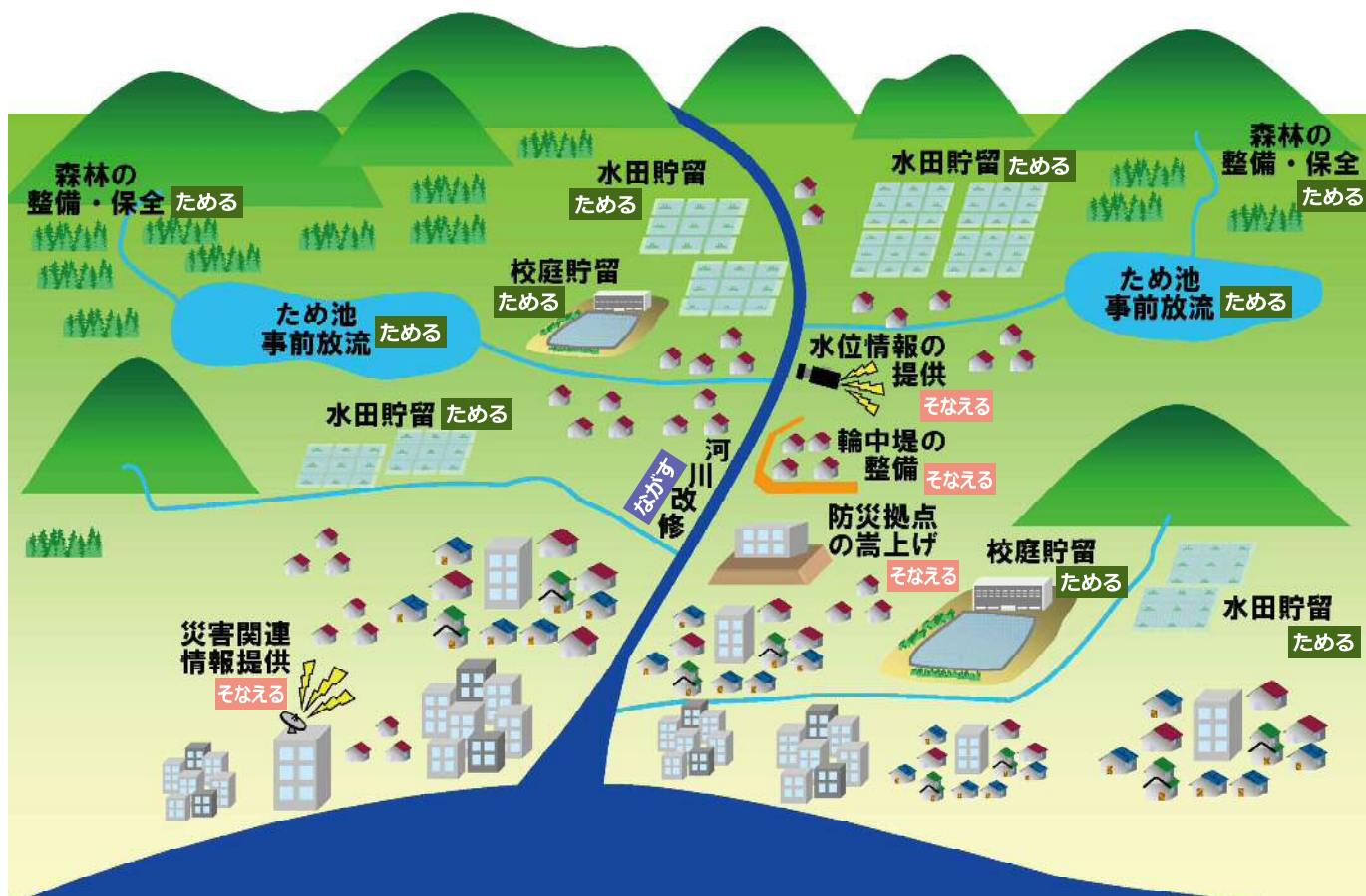
総合治水のイメージ図
